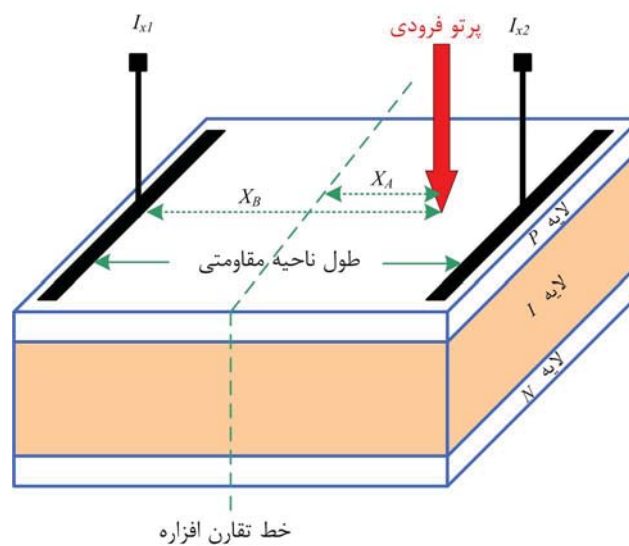
شکل (۱) نمای ساده از قسمتهای مختلف آشکارساز اثر جانبی. این ساختار برای حالت دو بعدی رسم شده است، اما برای سادگی، مختصات یک بعد در آن نشان داده شده است.
