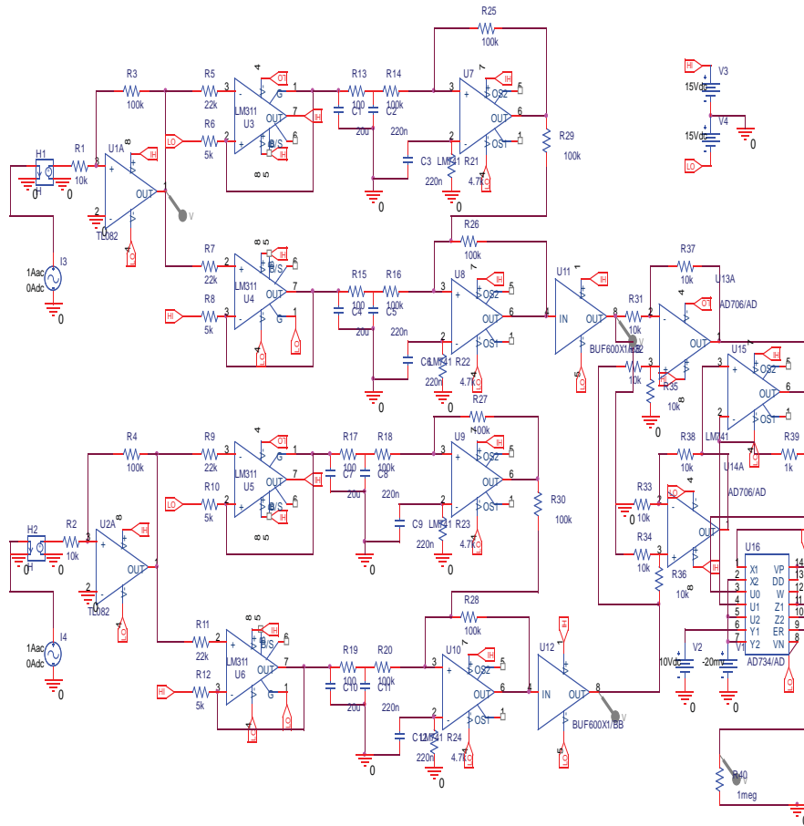
شکل (۴) مدار جانبی اصلاح شده آشکارساز اثر جانبی برای موقعیت X.
