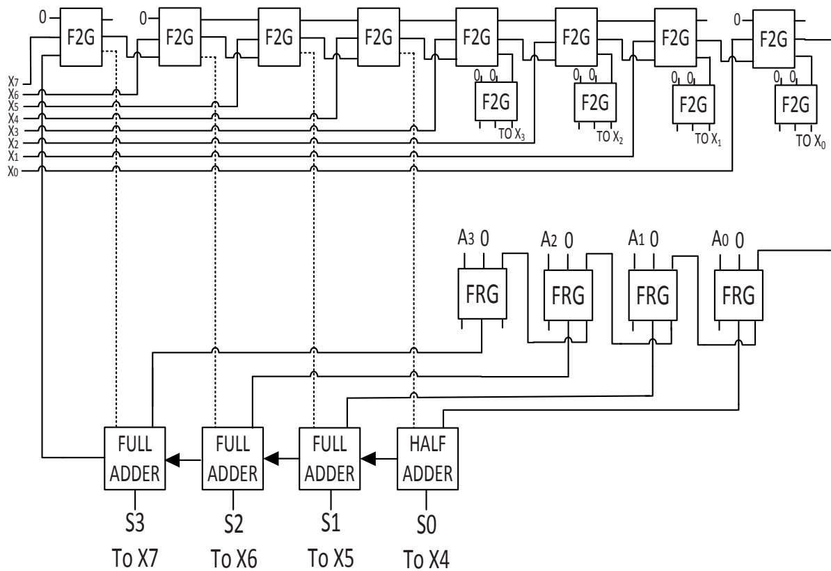
شکل ۱۸. مدار پیشنهادی برای ضرب‌کننده‌ی چهار بیتی بدون علامت تشخیص دهنده خطا مبتنی بر روش جمع و شیفت
