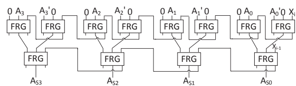
شکل ۹. مدار بخش مالتی‌پلکسرهای چهار به یک مطابق با [۱۷]
