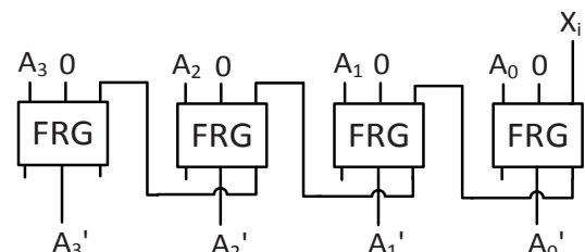
شکل ۱۶. مدار مالتی‌پلکسرهای دو به یک در ضرب‌کننده‌ی چهار بیتی پیشنهادی مبتنی بر روش جمع و شیفت
