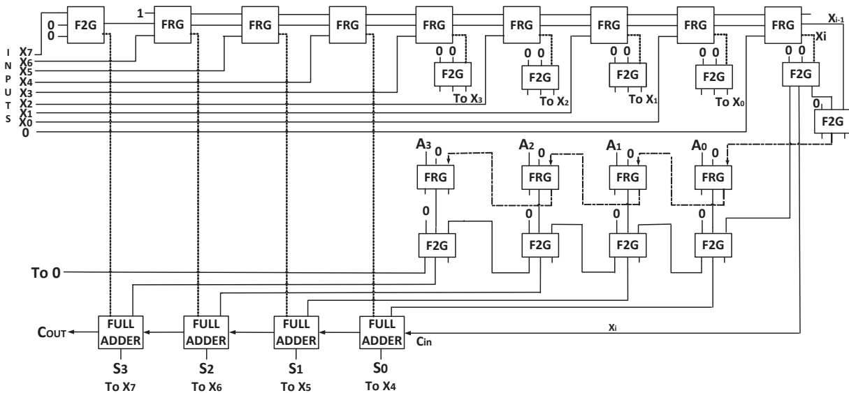
شکل ۱۱. ضرب‌کننده‌ی چهار بیتی مبتنی بر الگوریتم K ارائه شده در [۱۷]
