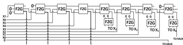
شکل ۱۲. مدار پیشنهادی بخش انتقال‌دهنده‌ی موازی در ضرب‌کننده‌ی چهار بیتی مبتنی بر روش بوث
