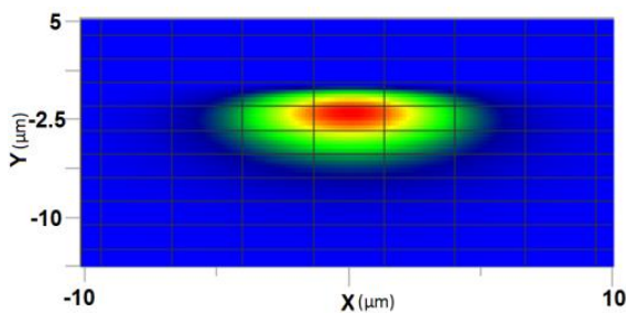
شکل ۱. عنوان مد نور موجبر با عرض ماسک ۶ μm تبادل پروتون یک ساعت در دمای ۱۷۰ درجه و آنیل ۵ ساعت در دمای ۳۷۵ درجه در طول موج ۱۵۵۰ nm.
