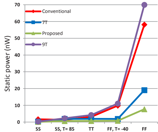
شکل ۱۶. توان استاتیک سلول ارائه شده، 9T، 7T، و سلول سنتی 6T در دماهای مختلف بر حسب سانتی‌گراد.
