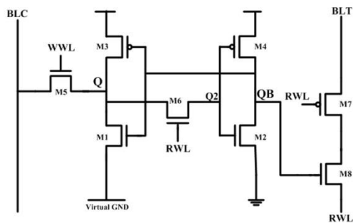
شکل ۵. شماتیک سلول ارائه شده.
