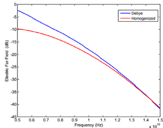
شکل ۸. میدان لایه نازک دبی با ضخامت سلول 0.5 mm در مقایسه با میدان حاصل از سلول همگن شده
