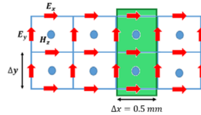
شکل ۷. شبکه FDTD حاوی لایه دبی با ضخامت t=0.5 \text{ mm} و اندازه سلول \Delta x = \Delta y = 0.5 \text{ mm}
