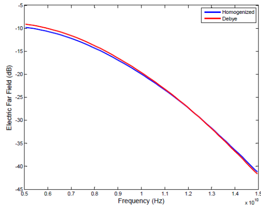
شکل ۹. میدان لایه نازک دبی با ضخامت سلول 0.1 mm در مقایسه با میدان حاصل از سلول همگن شده
