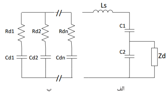
شکل ۳ الف. مولفه میدان الکتریکی در یک سلول شامل لایه نازک پاشنده از نوع دبابی (باتوجه به شکل ۱) ب. امدانس Z_{d(x)} شامل n قطب
