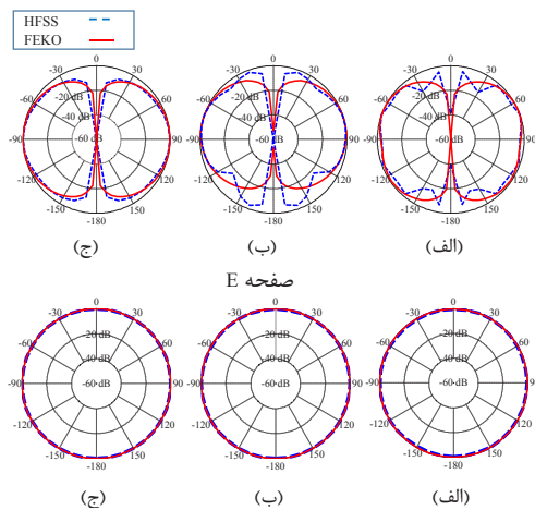
شکل ۶. الگوی تشعشی در فرکانس‌های الف (۱۸۵ MHz) ب (۳۵۴ MHz) ۵۲۳ MHz
