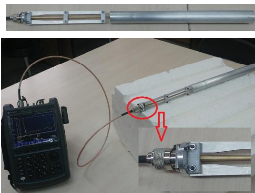
شکل ۱۰. نمونه آنتن پیشنهادی
