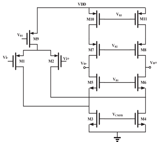
شکل ۱۴. آپامپ کسکود تا شده
