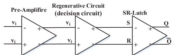
شکل ۱۵. بلوکی مقایسه کننده
