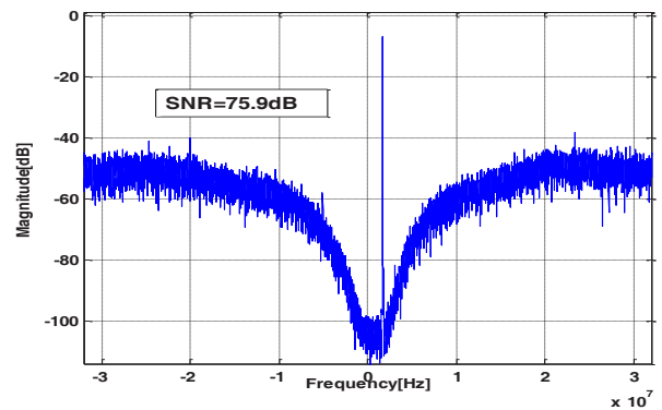
شکل ۱۸. طیف خروجی مدولاتور متعام پیشنهادی شبیه‌سازی شده در سطح ترانزیستور مد عملیاتی WCDMA
