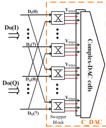
شکل ۸. بلوک DAC مختلط
