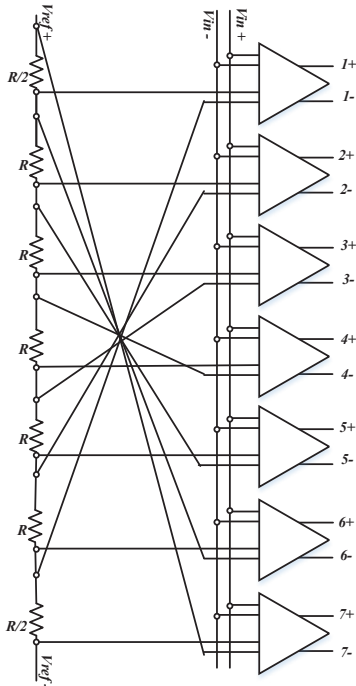
شکل ۱۶. ساختار بلوکی کوانتایزر ۳ بیتی
