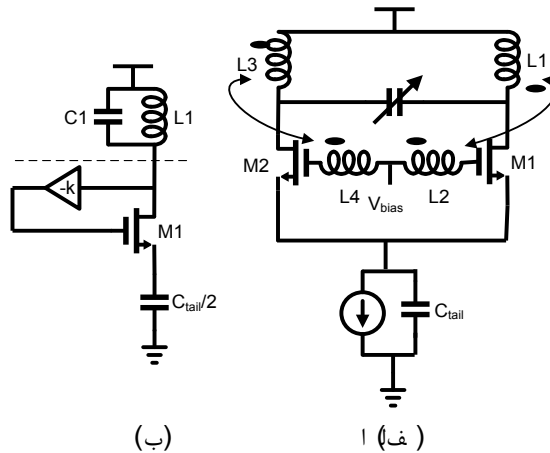
شکل ۱ الف) مدار یک ا (الف) بی‌تحقق یافته با ترا؛ (ب) نیم مدار اسیلاتور
