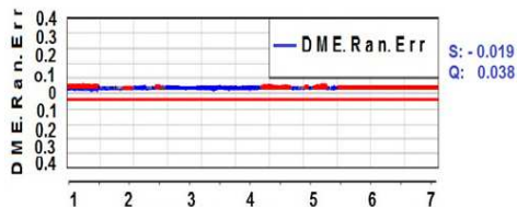
شکل ۲۳ ب. تعیین خطای فاصله هواپیما تا ایستگاه DME با ماهواره GPS
