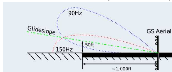
شکل ۱۶. سیگنال های عمودی برای تعیین شیب فرود هواپیما [۴]
