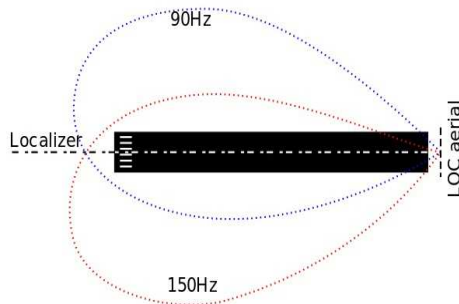
شکل ۱۲. پخش سیگنال‌های LLZ برای هدایت افقی هواپیما
