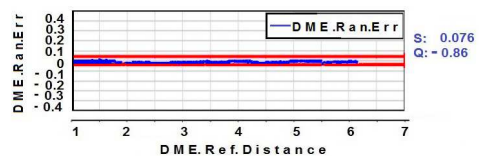
شکل ۲۷ ب. تعیین خطای فاصله هواپیما تا ایستگاه DME با DGPS
