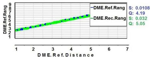
شکل ۲۳ الف. تعیین فاصله هواپیما تا ایستگاه DME با ماهواره GPS
