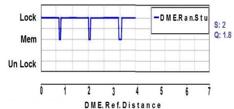
شکل ۲۶ ب. جستجوی موقعیت ایستگاه DME با GPS
