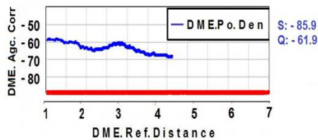
شکل ۲۴ ب. توان دریافتی هواپیما با ماهواره GPS
