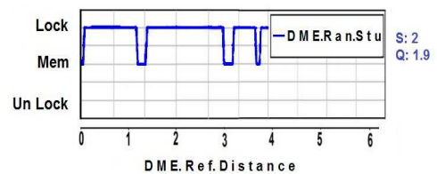
شکل ۲۶ الف. جستجوی موقعیت ایستگاه DME با روش DGPS
