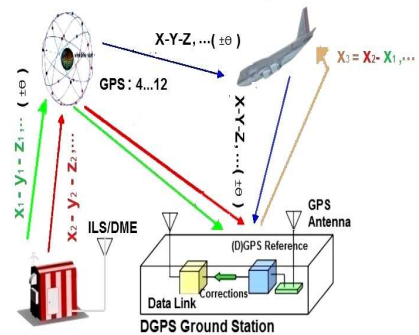
شکل ۱۱. اصلاح موقعیت هواپیما به کمک روش DGPS [۲۰]
