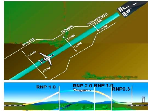
شکل ۹. بهبود پرواز با سرویس ناوبری RNP [۱۰].
