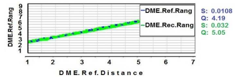
شکل ۲۷ الف. تعیین فاصله هواپیما تا ایستگاه DME با روش DGPS
