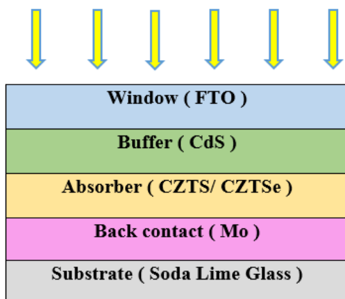
شکل ۱. ساختار سلول خورشیدی CZTS/CZTSe
