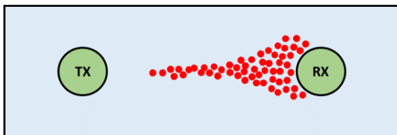
شکل ۱۳. دم بلند تشکیل شده از مولکول‌ها در انتقال یک بیت "۱" که منجر به وقوع ISI در مخابرات مولکولی می‌شود
