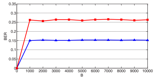
شکل ۱۶. تاثیر تعداد بیت‌های ارسالی بر روی میزان نرخ خطای بیت با حذف ISI فقط از یک بیت بعدی بعد از آخرین بیت "۱" دریافتی همچنین در شکل ۱۷، میزان ISI از دو بیت بعدی، بعد از آخرین بیت "۱" دریافتی کم شده است. در این شکل نرخ خطای بیت در حدود ۰/۰۸ است. نرخ خطای بیت به میزان قابل توجهی کم شده است ولی هنوز هم نیاز به بهبود حس می‌شود.
