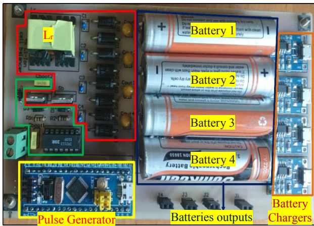
شکل ۱۶. تصویر نمونه‌ی آزمایشگاهی مدار ساخته شده با چهار باتری لیتیوم-یونی سری شده
