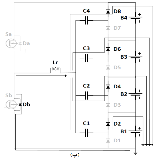
شکل ۳. مدار معادل های وضعیت های کاری مختلف مبدل پیشنهادی در یک دوره تناوب کلیدزنی در حالت مساوی بودن ولتاژ باتری ها
