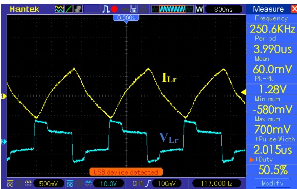
شکل ۲۱. شکل موج های ولتاژ و جریان سلف L_r
