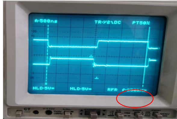
شکل ۱۸. شکل موج ولتاژهای گیت-سورس MOSFET ها
