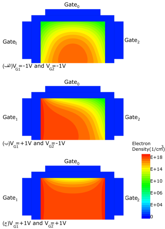
شکل ۶. توزیع چگالی الکترون ها در وسط کانال از نمای جانبی زمانیکه V_{G0}=-1V و V_{DS}=2V باشد تحت شرایط الف) V_{G1}=-1V و V_{G2}=-1V (ب) V_{G1}=+1V و V_{G2}=-1V (ج) V_{G1}=+1V و V_{G2}=+1V
