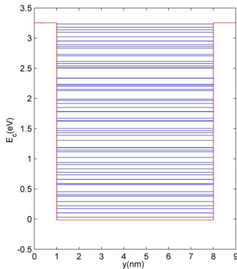
شکل ۳. نوار انرژی باند هدایت در وسط کانال و در راستای عمق افزاره y در حالت بدون بایاس.
