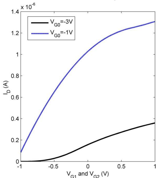
شکل ۴. منحنی جریان درین برحسب ولتاژ ورودی با فرض V_{G1}=V_{G2} ، در دو حالت V_{G0}=-3V و V_{G0}=-1V . در هر دو منحنی V_{DS}=+2V می باشد
