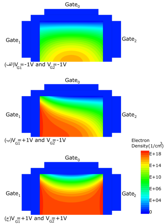
شکل ۵. توزیع چگالی الکترون ها در وسط کانال از نمای جانبی زمانیکه V_{G0}=-3V و V_{DS}=2V باشد تحت شرایط الف) V_{G1}=-1V و V_{G2}=-1V (ب) V_{G1}=+1V و V_{G2}=-1V (ج) V_{G1}=+1V و V_{G2}=+1V
