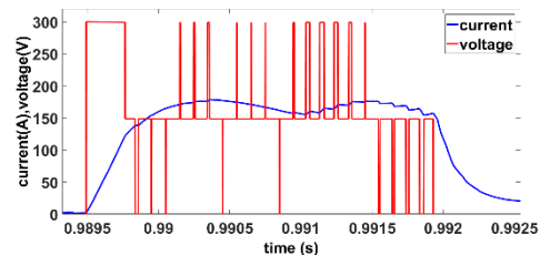
ب) روش PPWM سرعت ۲۰۰۰ RPM - ریپل پیک تا پیک ۵.۲ آمپر
