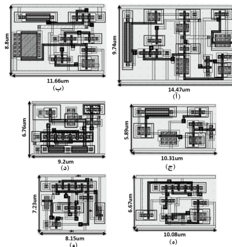
شکل ۹. طرح Layout ساختارهای ارائه شده در (آ) [۷] 140/93 میکرومتر مربع، (ب) [۲۲] 102/61 میکرومتر مربع، (ج) [۱] 60/73 میکرومتر مربع، (د) [۲۳] 62/2 میکرومتر مربع، (ه) [۸] 67/23 میکرومتر مربع، (و) مبدل پیشنهادی 59/1 میکرومتر مربع.
