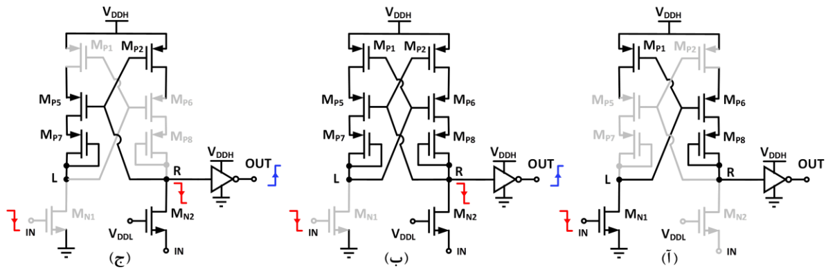
شکل ۴. مراحل عملکرد مدار پیشنهادی هنگام گذار پایین‌رونده ورودی.
