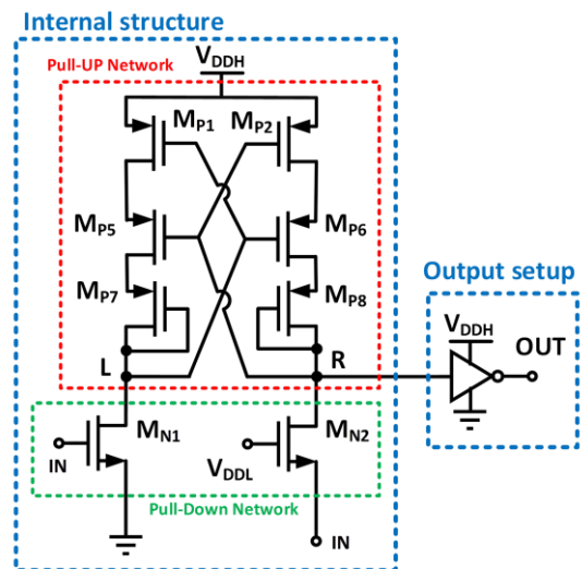
شکل ۳. طرح اولیه ساختار پیشنهادی.
