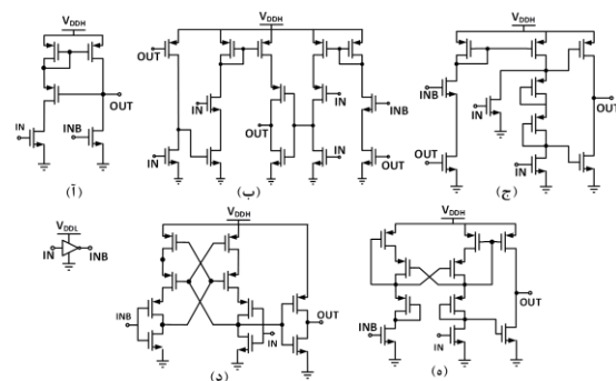
شکل ۸. معماری‌های ارائه شده در (آ) [۱]، (ب) [۷]، (ج) [۲۲]، (د) [۲۳]، (ه) [۲۳].
