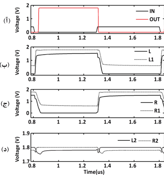
شکل ۷. شکل موج ولتاژ گره‌های داخلی مبدل پیشنهادی.
