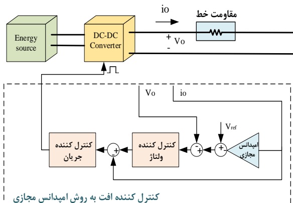
شکل ۲. بلوک دیاگرام کنترل کننده افت به روش امپدانس مجازی
