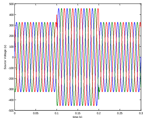
شکل (۴- الف). شکل موج ولتاژ منبع (بیشود ولتاژ)
