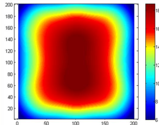
شکل ۸. توزیع دامنه میدانی الکتریکی بر روی سطح بازتابنده اصلی
