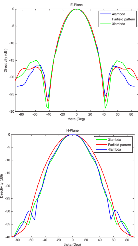
شکل ۶ بررسی تغییر فاصله بین پروب و AUT بر الگوی میدان دور صفحه‌های E و H آنتن تحت آزمایش در فرکانس 10GHz
