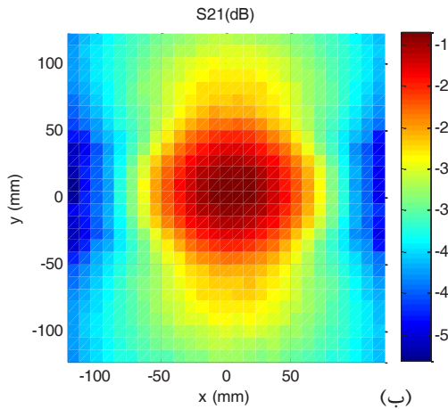
شکل ۸. اندازه‌ی کوپلاژ بین پروب و AUT در نقاط مختلف روی صفحه (الف) ابعاد صفحه 8\lambda \times 8\lambda (ب) ابعاد صفحه 16\lambda \times 16\lambda
