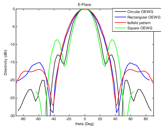
شکل ۲: مقایسه‌ی الگوی میدان دور بدست آمده از مدلسازی اندازه‌گیری با سه نوع پروب مختلف OEWG در فرکانس ۱۰GHz
