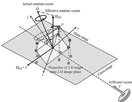
شکل ۵. صفحه انعکاس تصویر در ISAS [۲۶]
