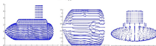
شکل ۱۲. نماهای مختلف از مدل در نظر گرفته شده برای زیردریایی هدف
