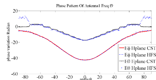
شکل ۳۱. رفتار پترن فاز آنتن ۱ در دو نرم افزار CST و HFSS در فرکانس ۹ گیگاهرتز (f 9 )
