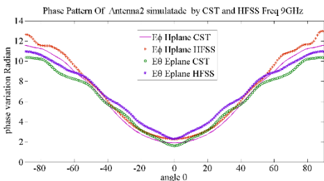
شکل ۳۵. رفتار پترن فاز آنتن ۲ در دو نرم افزار CST و HFSS در فرکانس ۹ گیگاهرتز (f 9 )
