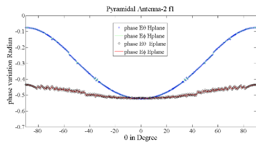
شکل ۱۶. رفتار فاز آنتن ۲ در فرکانس f_1
