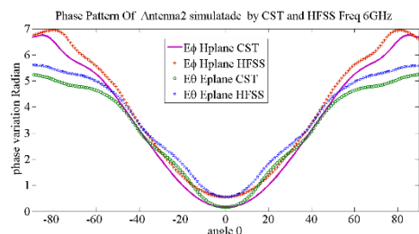
شکل ۳۴. رفتار پترن فاز آنتن ۲ در دو نرم افزار CST و HFSS در فرکانس ۶ گیگاهرتز (f 6 )
