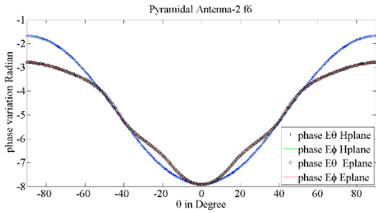
شکل ۱۸. رفتار فاز آنتن ۲ در فرکانس f_6
