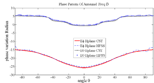
شکل ۲۹. رفتار پترن فاز آنتن ۱ در دو نرم افزار CST و HFSS در فرکانس ۳ گیگاهرتز (f 3 )
