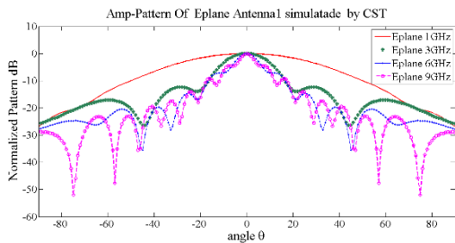
شکل ۲۴. رفتار پترن دامنه آنتن ۱ صفحه الکتریکی شبیه‌سازی شده در CST
