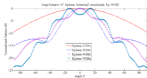
شکل ۲۲. رفتار پترن دامنه آنتن ۲ صفحه الکتریکی شبیه‌سازی شده در HFSS
