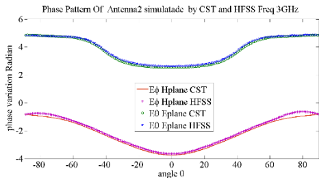
شکل ۳۳. رفتار پترن فاز آنتن ۲ در دو نرم افزار CST و HFSS در فرکانس ۳ گیگاهرتز (f 3 )
