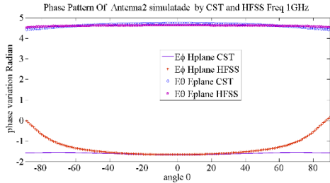
شکل ۳۲. رفتار پترن فاز آنتن ۲ در دو نرم افزار CST و HFSS در فرکانس ۱ گیگاهرتز (f 1 )
