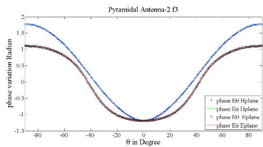
شکل ۱۷. رفتار فاز آنتن ۲ در فرکانس f_3
