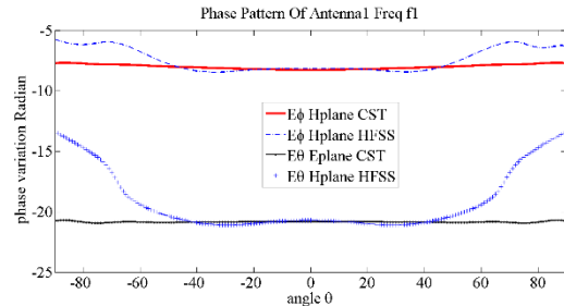
شکل ۲۸. رفتار پترن فاز آنتن ۱ در دو نرم افزار CST و HFSS در فرکانس ۱ گیگاهرتز (f 1 )
