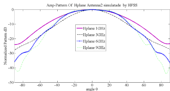
شکل ۲۳. رفتار پترن دامنه آنتن ۲ صفحه مغناطیسی شبیه‌سازی شده در HFSS
