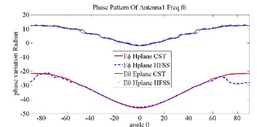
شکل ۳۰. رفتار پترن فاز آنتن ۱ در دو نرم افزار CST و HFSS در فرکانس ۶ گیگاهرتز (f 6 )
