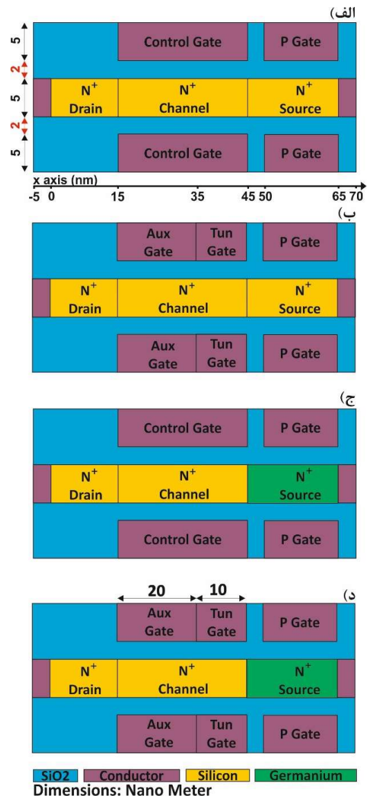
شکل ۱. تصویر توصیفی دو بعدی الف) SMG-JLTFET (ب) DMG-JLTFET (ج) SMG-H-JLTFET (د) DMG-H-JLTFET
